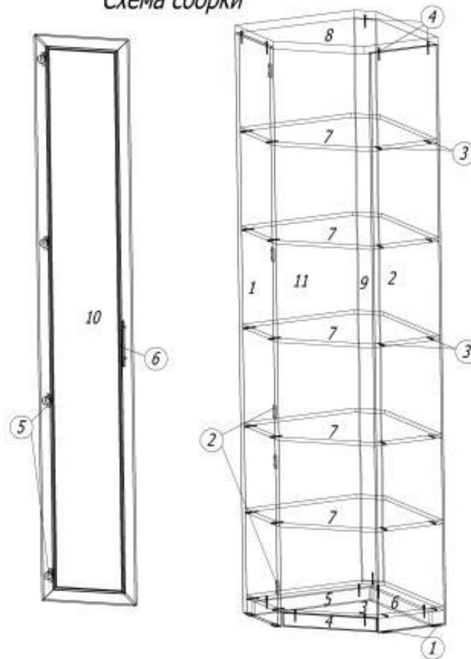
Схема сборки
